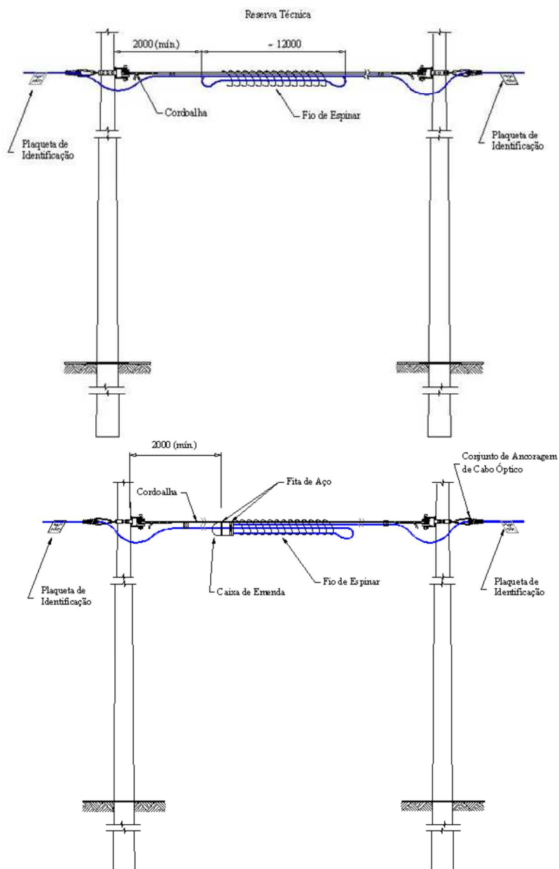
Figura 3: Padrão de instalação no vão entre os postes.
